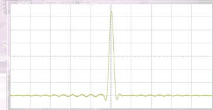
Das gleiche Signal wiedergegeben mit MDAT: Per DSP ans Signal angepasste Filtertypen reduzieren Vor- und Nachschwingen deutlich.
