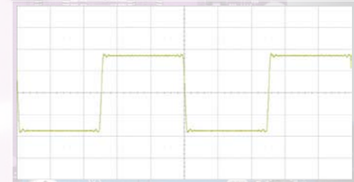
In MDAT-Wiedergabe verläuft das Dach bei Rechteckschwingungen nahezu linear und mit deutlich geringeren Verformungen.
