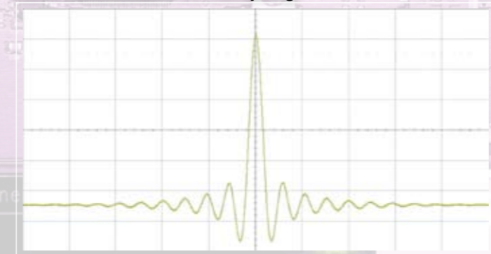
Wiedergabe eines Nadelimpulses (Diracstoß): Oversampling mit FIR-Filtern erzeugt sichtbares Vor- und Nachschwingen.
