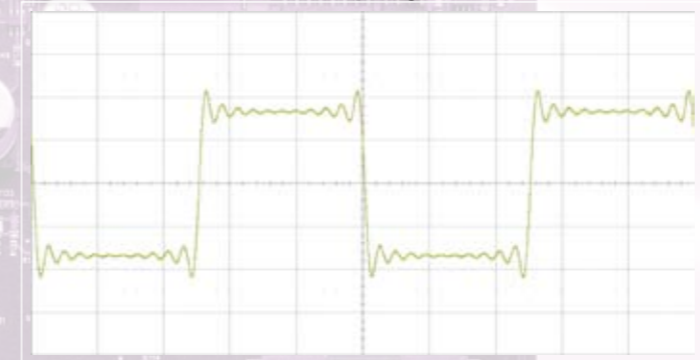
Auch bei Rechteck-Signalen zeigt sich mit gängigem Oversampling ein deutlich sichtbares „Ringing“.
