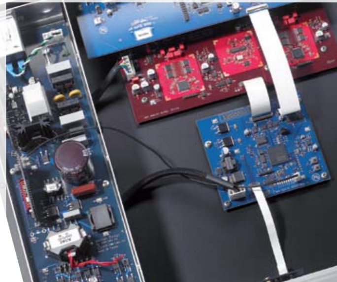
Alles aus eigener Hand: Statt auf Wandlerelektronik von der Stange setzt der MA 1 auf Meitner-exklusive Schaltungstechnik.
